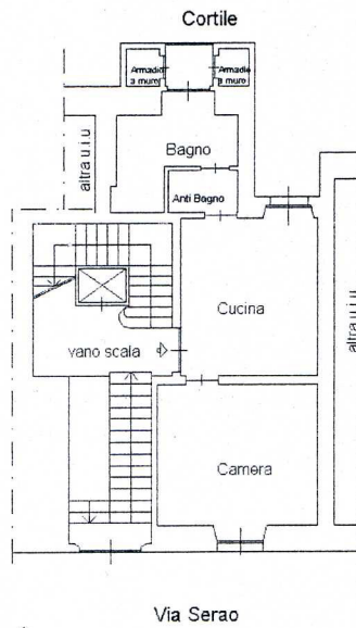
Piano Primo - Ammezzato (h. 3.20 m)
